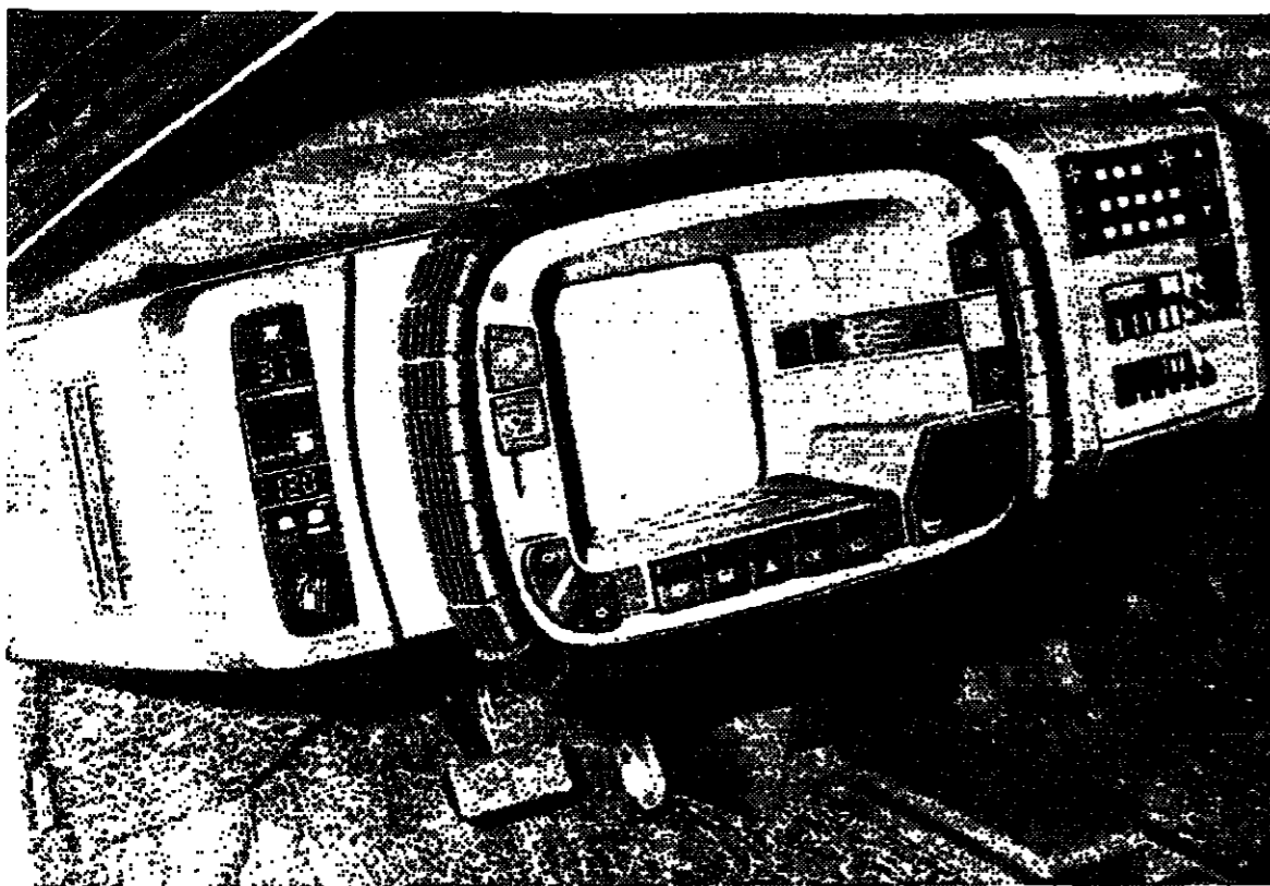
Mazda experimentiert mit einer Cockpitstudie, in der ein sogenannter Lenkkranz den Bildschirm des Leitsystems umschließt. Statt ein Lenkrad zu drehen, steuert der Fahrer das Fahrzeug mit leichtem Fingerdruck auf Kontaktelemente und hat freie Sicht auf den Bildschirm (links). - Bisher erprobt: Straßenplan und Gebietskarte auf einem Bildschirm in konventioneller Anordnung auf der Konsole (rechts).
